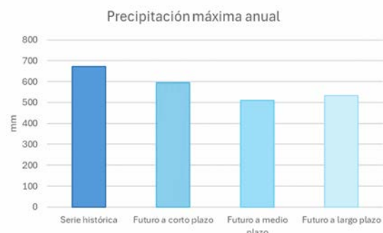
Figura 40. Diagramas de variación de los valores de precipitación media (izquierda) y máxima (derecha) anuales en Guadalcanal para la serie histórica de 1961 a 1990 y para los horizontes temporales de futuro a corto, medio y largo plazo.
