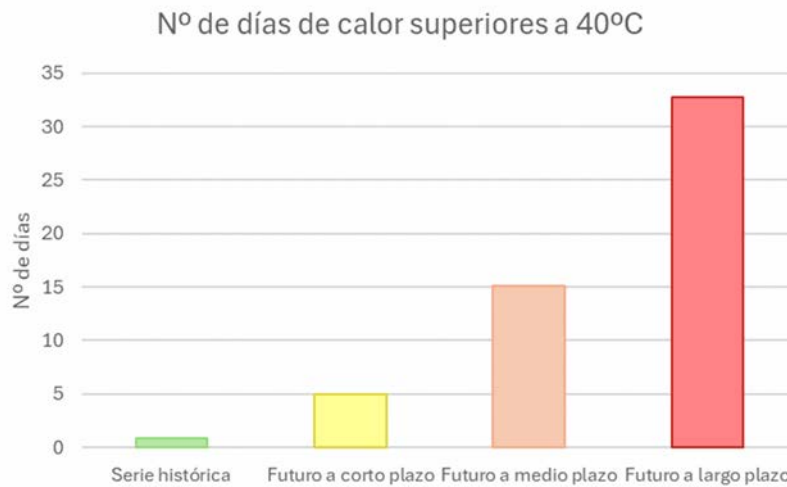
Figura 39. Diagrama de variación del número de días en los que se superan los 40°C al año en Guadalcanal para la serie histórica de 1961 a 1990 y para los horizontes temporales de futuro a corto, medio y largo plazo.
