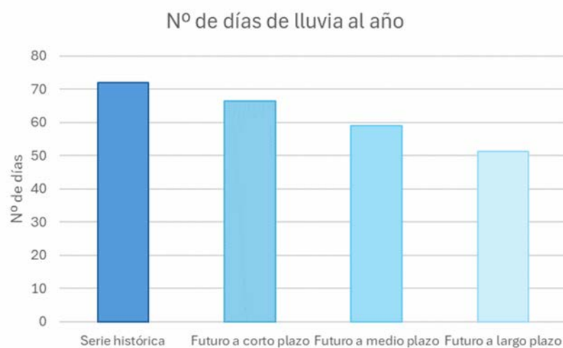
Figura 41. Diagrama de variación del número de días al año en los que llueve en Guadalcanal para la serie histórica de 1961 a 1990 y para los horizontes temporales de futuro a corto, medio y largo plazo.
