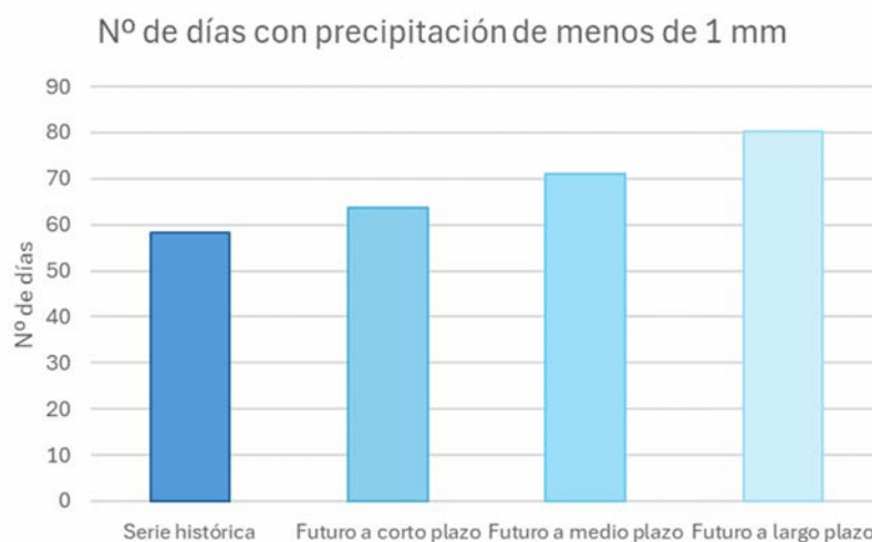
Figura 42. Diagrama de variación del número de días al año en los que se registran en Guadalcanal valores de precipitación inferiores a 1 mm para la serie histórica de 1961 a 1990 y para los horizontes temporales de futuro a corto, medio y largo plazo.
