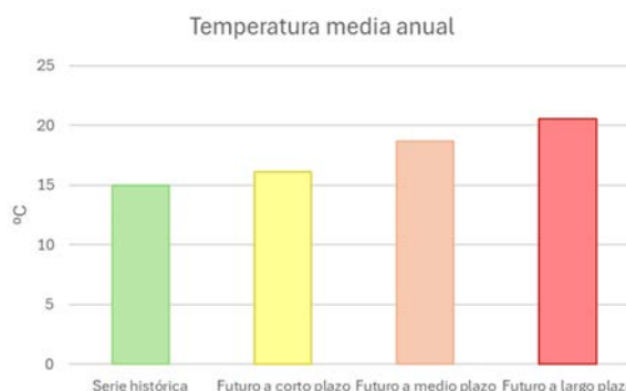
Figura 38. Diagramas de variación de las temperaturas media (izquierda) y máximas (derecha) anuales en Guadalcanal para la serie histórica de 1961 a 1990 y para los horizontes temporales de futuro a corto, medio y largo plazo.
