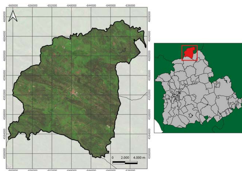
Figura 3. Ortofoto y situación geográfica de Guadalcanal respecto a la provincia de Sevilla.
