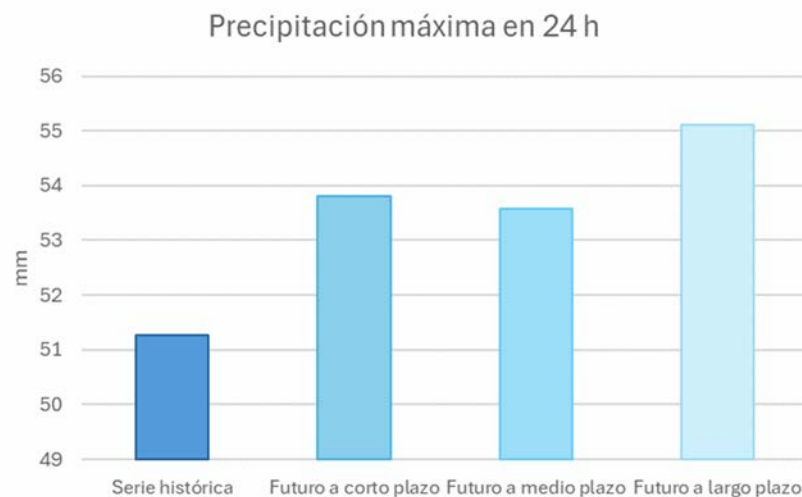
Figura 43. Diagrama de variación de los valores de precipitación máxima en 24 h en Guadalcanal para la serie histórica de 1961 a 1990 y para los horizontes temporales de futuro a corto, medio y largo plazo.
