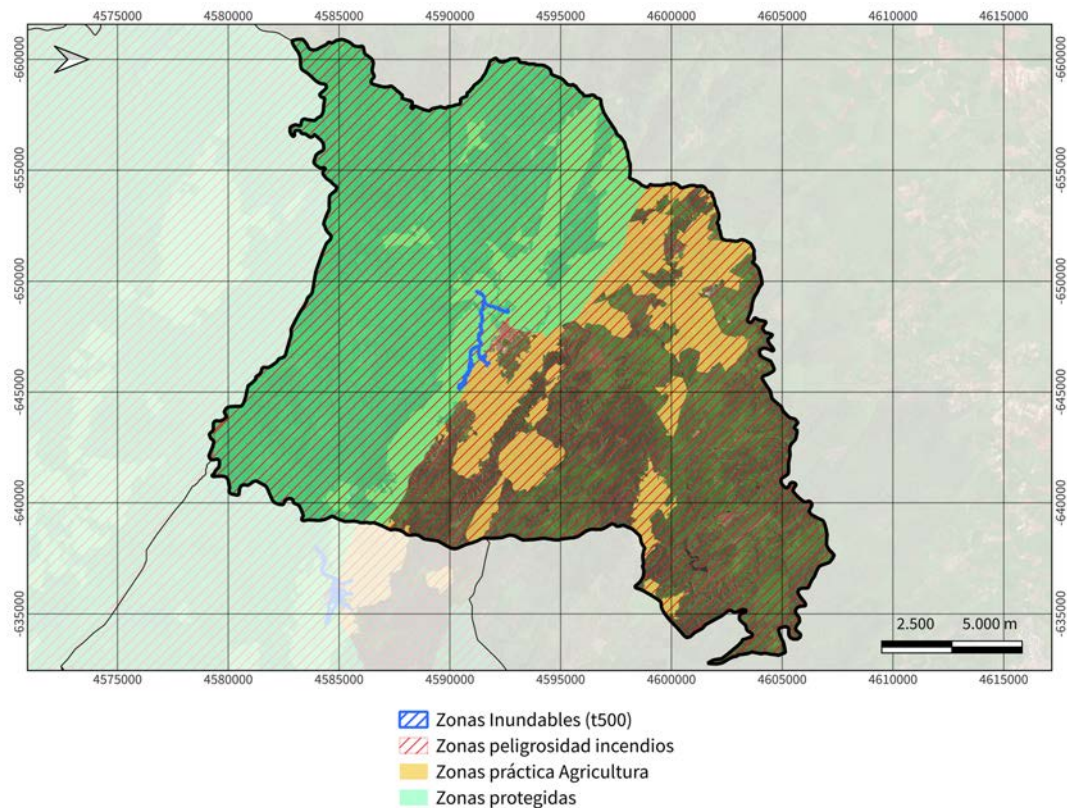
Figura 44. Mapa de las Zonas Especialmente Vulnerables de Guadalcanal.
