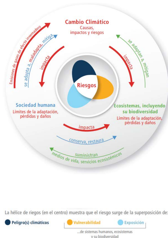
Figura 37. Cambio Climático: esquema de causas, impactos y riesgos.
